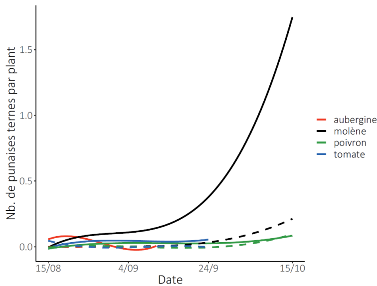
Figure 1. Prédiction de la variation des populations de punaises ternes (lignes pleines) et de Nabis (ligne pointillée) de la mi-août à la mi-octobre sur quatre plantes hôtes (molène, aubergine, poivron et tomate).
